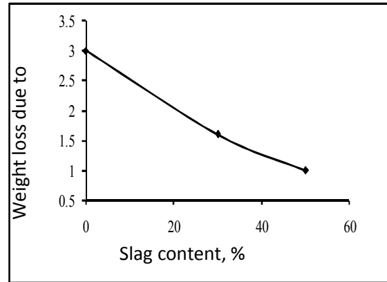
Fig. 2. CH of OPC/slag pastes
